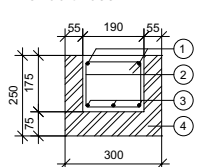
Překlad tl. 300 mm
