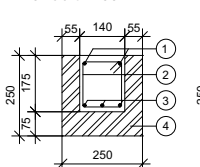
Překlad tl. 250 mm
