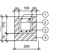
Překlad tl. 200 mm
