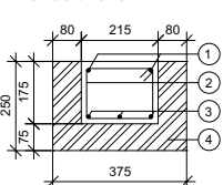
Překlad tl. 375 mm
