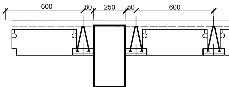
vsadený nosník do stropu
