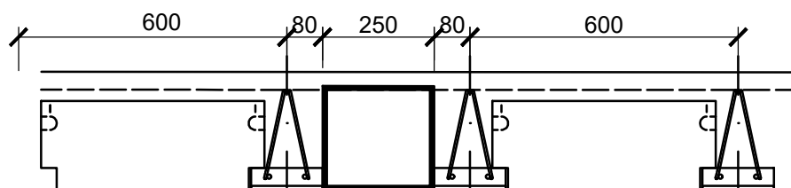
obrátенý nosník zapustený do stropu
