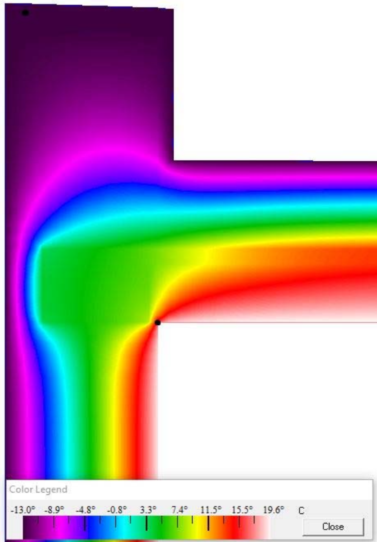
Pribeh teplôt konštrukciu - vykreslenie pomocou teplotného poľa
