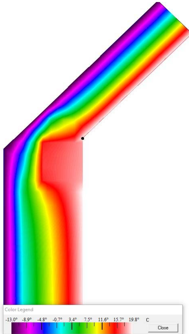
Priebeh teplôt konštrukciou - vykreslenie pomocou teplotného poľa
