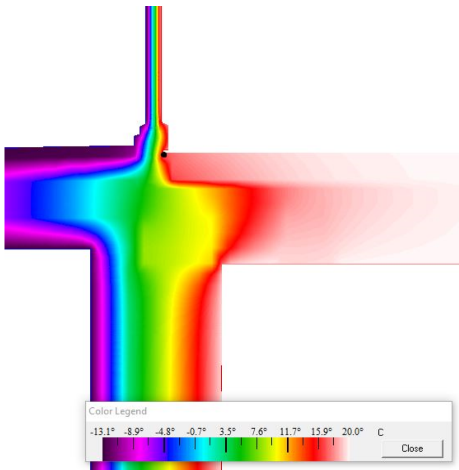
Pribeh teplôt konštrukciou - vykreslenie pomocou teplotného poľa
