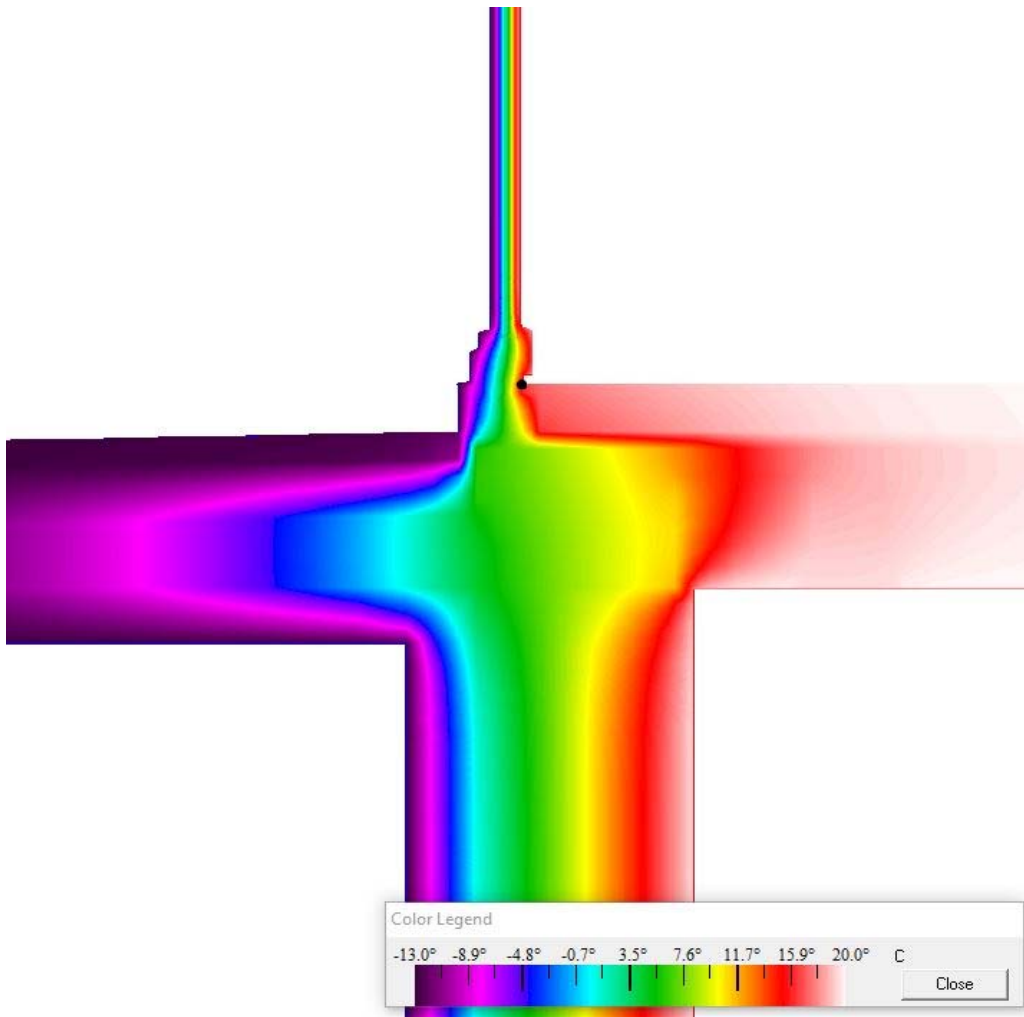
Pribeh teplôt konštrukciou - vykreslenie pomocou teplotného poľa
